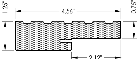
1 COMPOSITE JAMB
