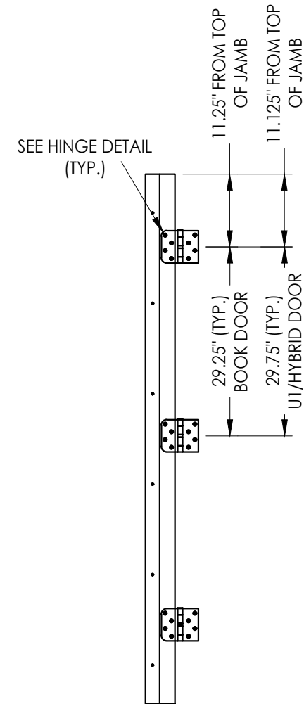
HINGE JAMB
